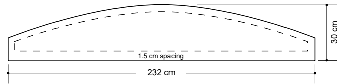
Header - QTY1
